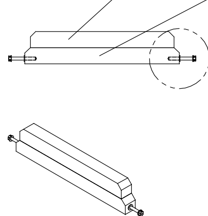
Hinter-Achse, 1x
