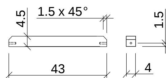
Achsteil, 1x
