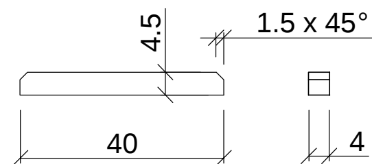
Achsteil, 1x
